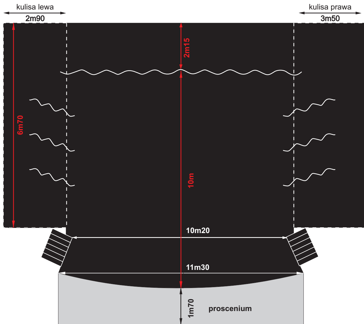
WYMIARY SCENY Miejskiego Domu Kultury w Radomsku
